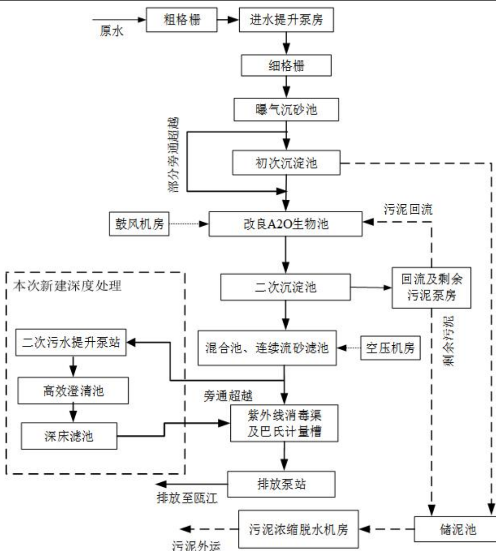
图 4-1 污水处理工艺流程示意图
