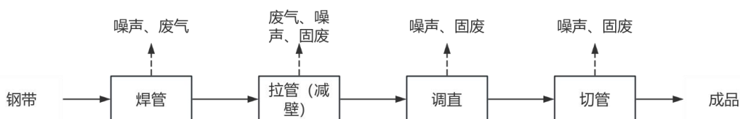
图 2-1 生产工艺流程及产污环节示意图
